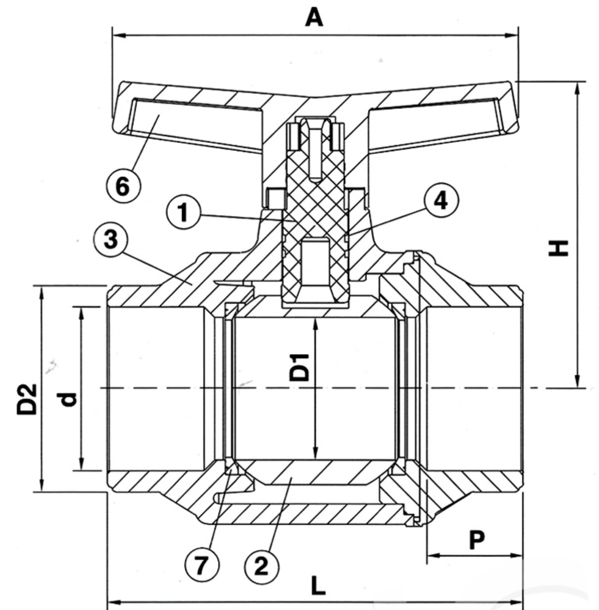
DN65~DN150
